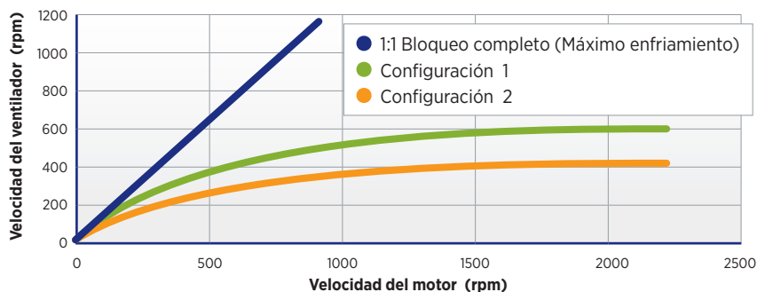
RENDIMIENTO DEL EMBRAGUE VENTILADOR DUROSPEED K32 Velocidad de ralentí se ajusta a la medida según el tipo de aplicación
